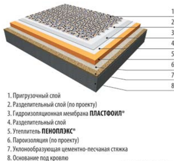
Рис. 2. Балластная кровля с материалом ПЛАСТФОИЛ®
