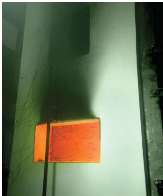
Рис. 2. Теплоизоляционная система с тонким штукатурным слоем ПЕНОПЛЭКС® Фасад после испытаний
